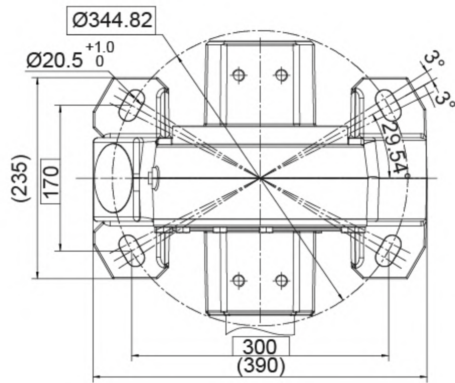
TOP VIEW 俯视图
