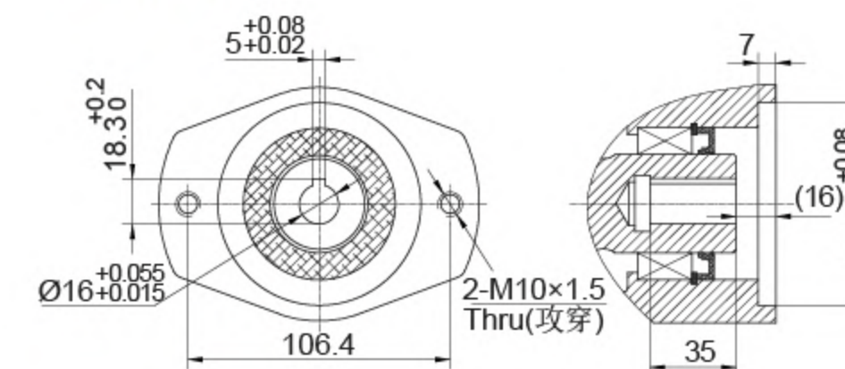
VIEW B B向视图
