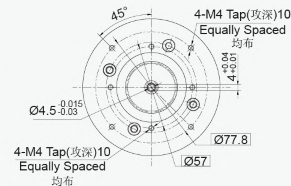
VIEW P OPTION P向选项
