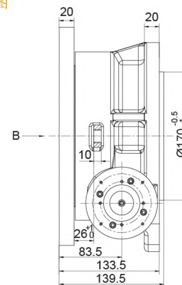
TOP VIEW 俯视图
