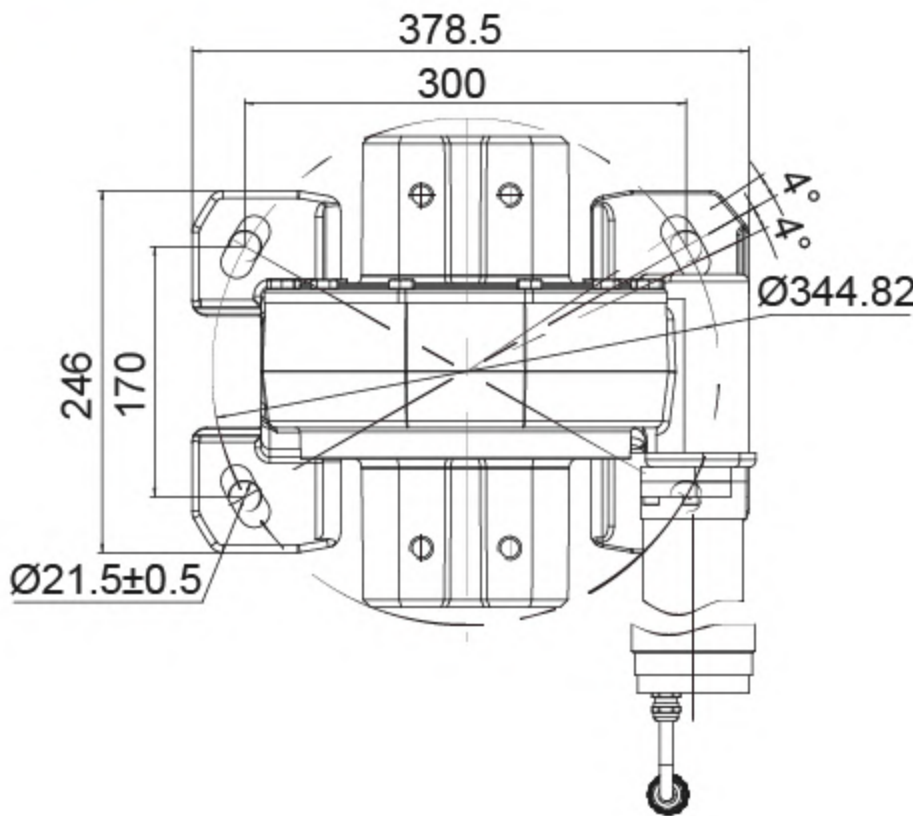
TOP VIEW 俯视图
