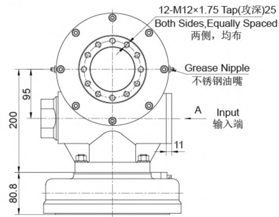
FRONT VIEW 正视图
