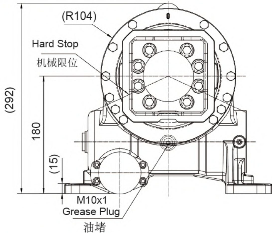
FRONT VIEW 正视图
