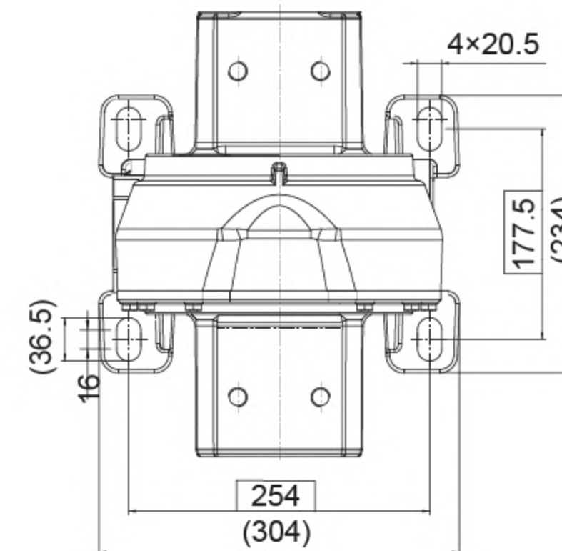
TOP VIEW 俯视图
