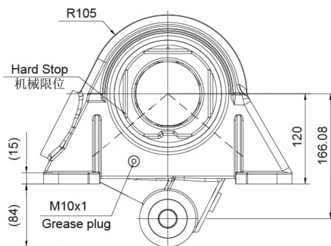
FRONT VIEW 正视图
