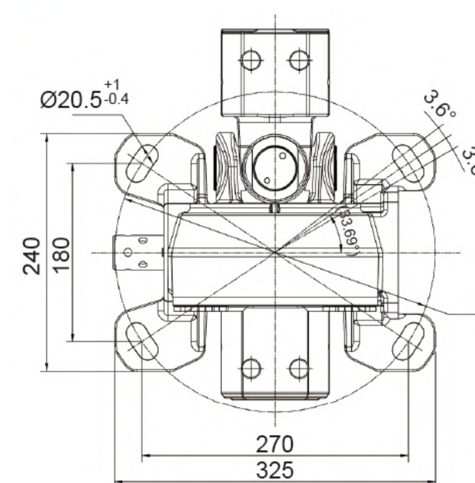
TOP VIEW 俯视图
