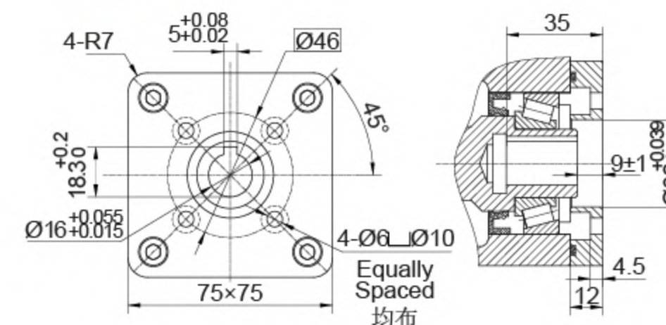
VIEW B B向视图
