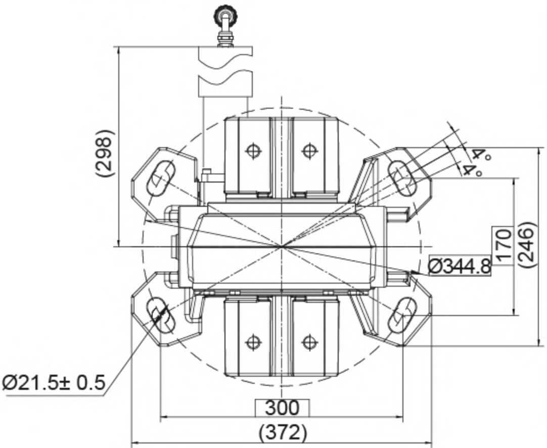
TOP VIEW 俯视图
