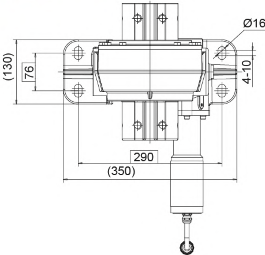
TOP VIEW 俯视图
