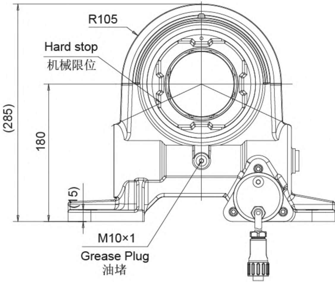
FRONT VIEW 正视图
