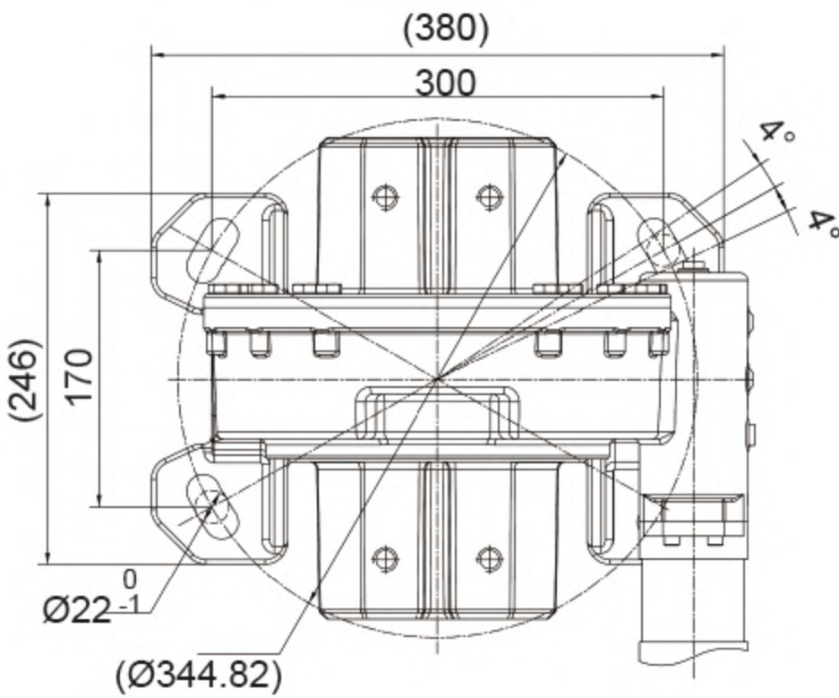
TOP VIEW 俯视图
