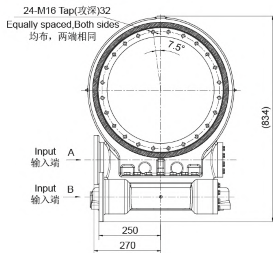
FRONT VIEW 正视图
