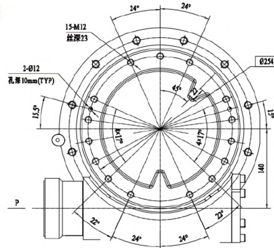
FRONT VIEW 正视图
