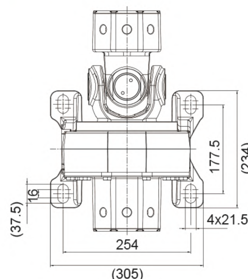
TOP VIEW 俯视图
