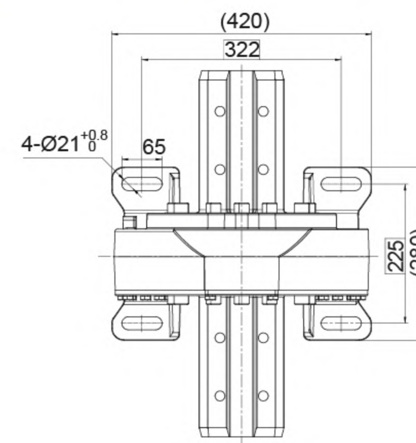
TOP VIEW 俯视图
