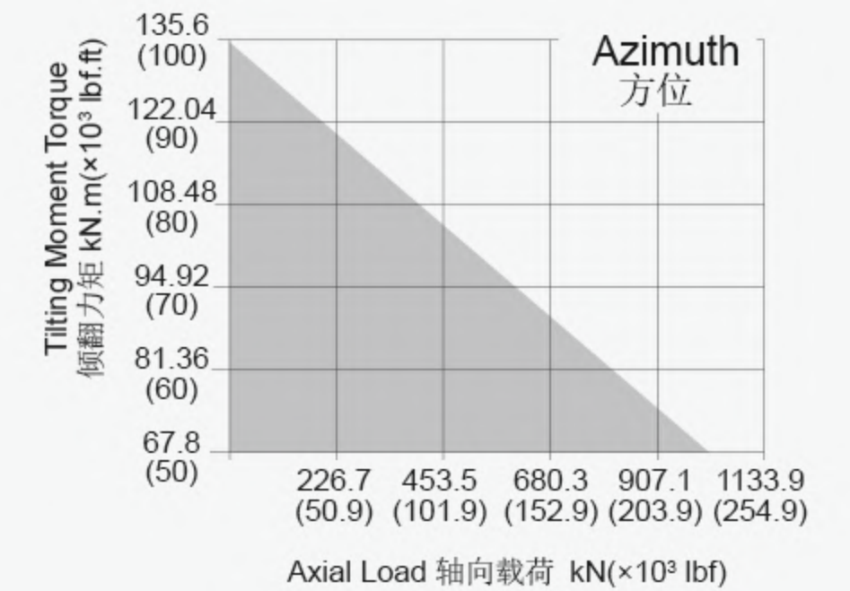
MOMENT LOAD CHART 承载力矩图
