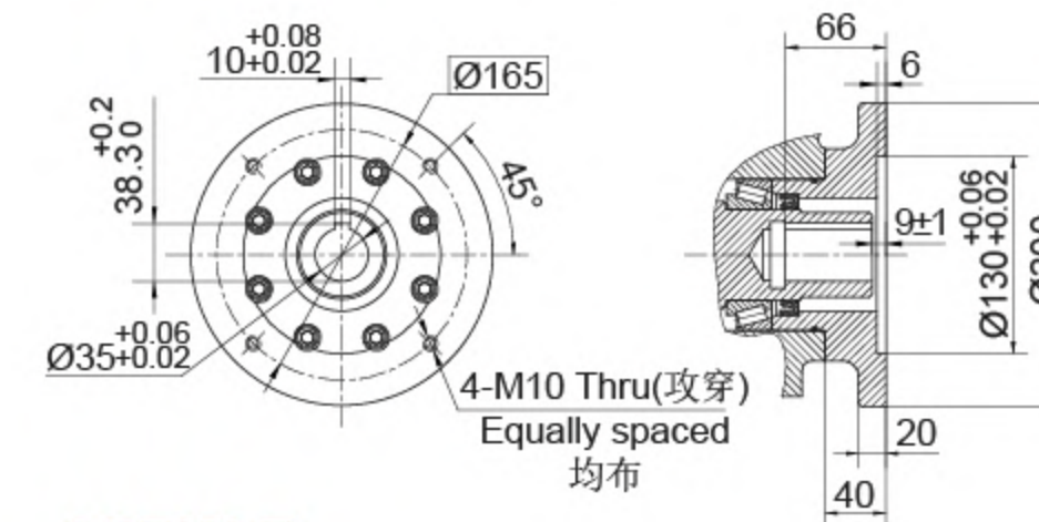
VIEW B B向视图
