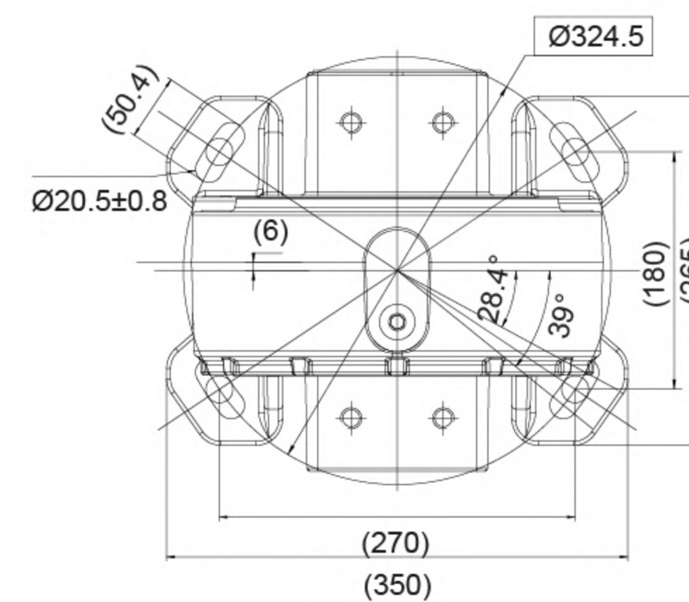
TOP VIEW 俯视图
