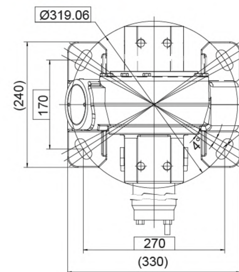
TOP VIEW 俯视图
